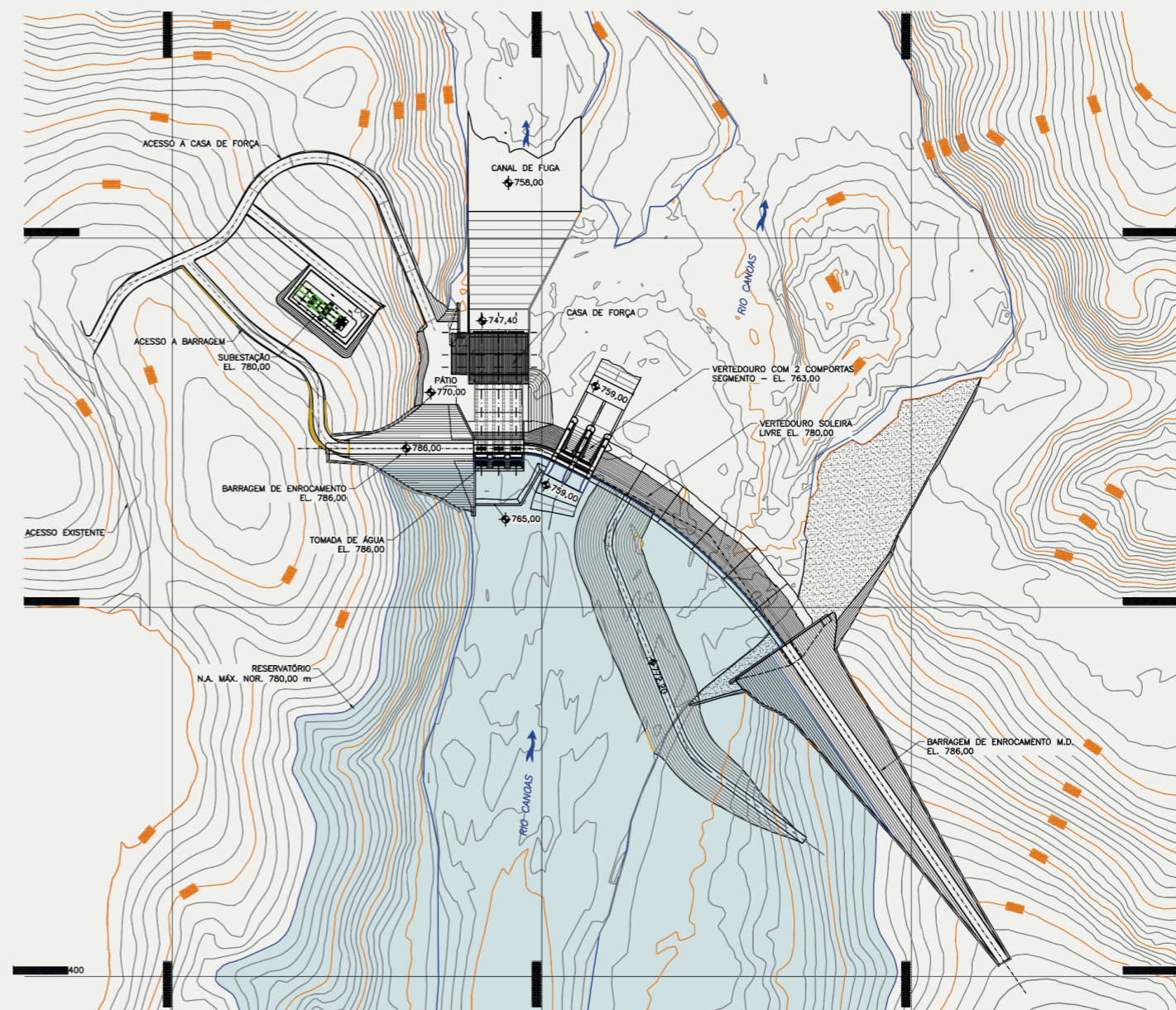
Arranjo da PCH Canoas.
