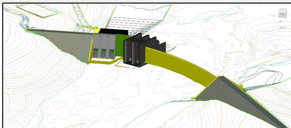
Arranjo geral da PCH Canoas - vista de montante.
