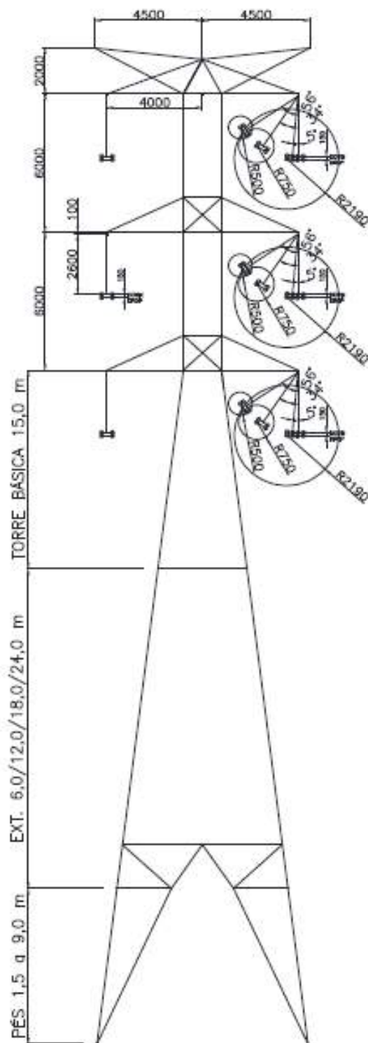
Figura 6.3-9: Silhueta da estrutura N2DSL1/N2DES2 (Torre de Ancoragem Suspensão Estaiada Leve) - LT de 230 kV.
