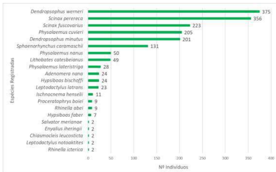
Gráfico 10.1-12: Número de registros por espécies da herpetofauna registrada na área de influência do empreendimento.
