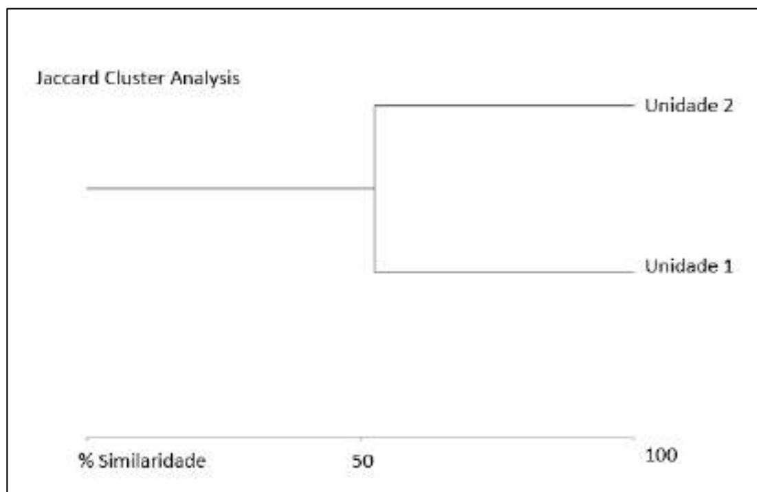
Gráfico 10.1-21: Análise de Agrupamento (Índice de Jaccard) para a composição de espécies entre as unidades amostrais durante o levantamento de aves na área de influência da LT 525/230 kV Rio do Sul – Indaial – Gaspar II (campanha do verão e outono de 2019).
