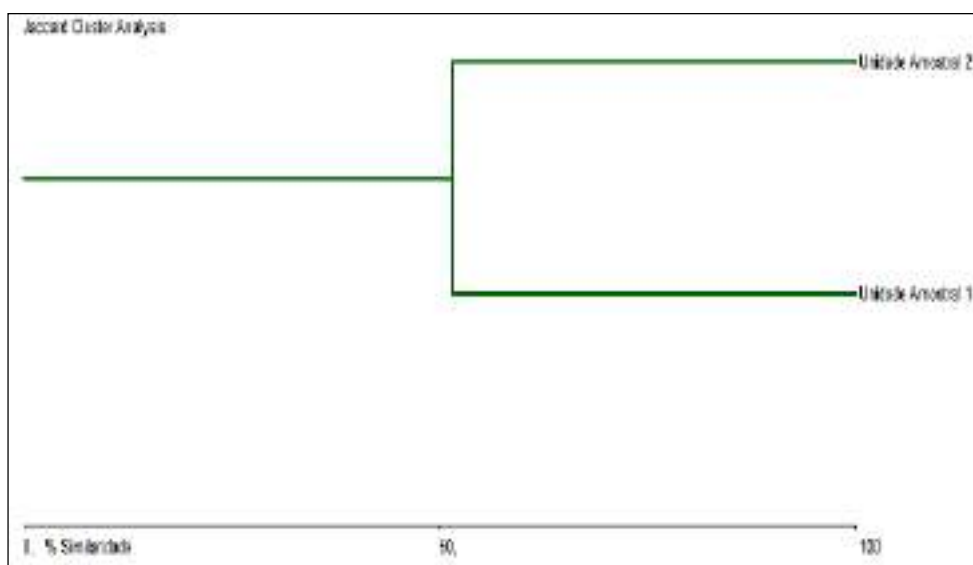
Gráfico 10.1-14: Análise de Agrupamento (Índice de Jaccard) para a composição de espécies entre as unidades amostrais durante o levantamento de anfíbios e répteis na área de influência (campanhas de verão e outono de 2019).
