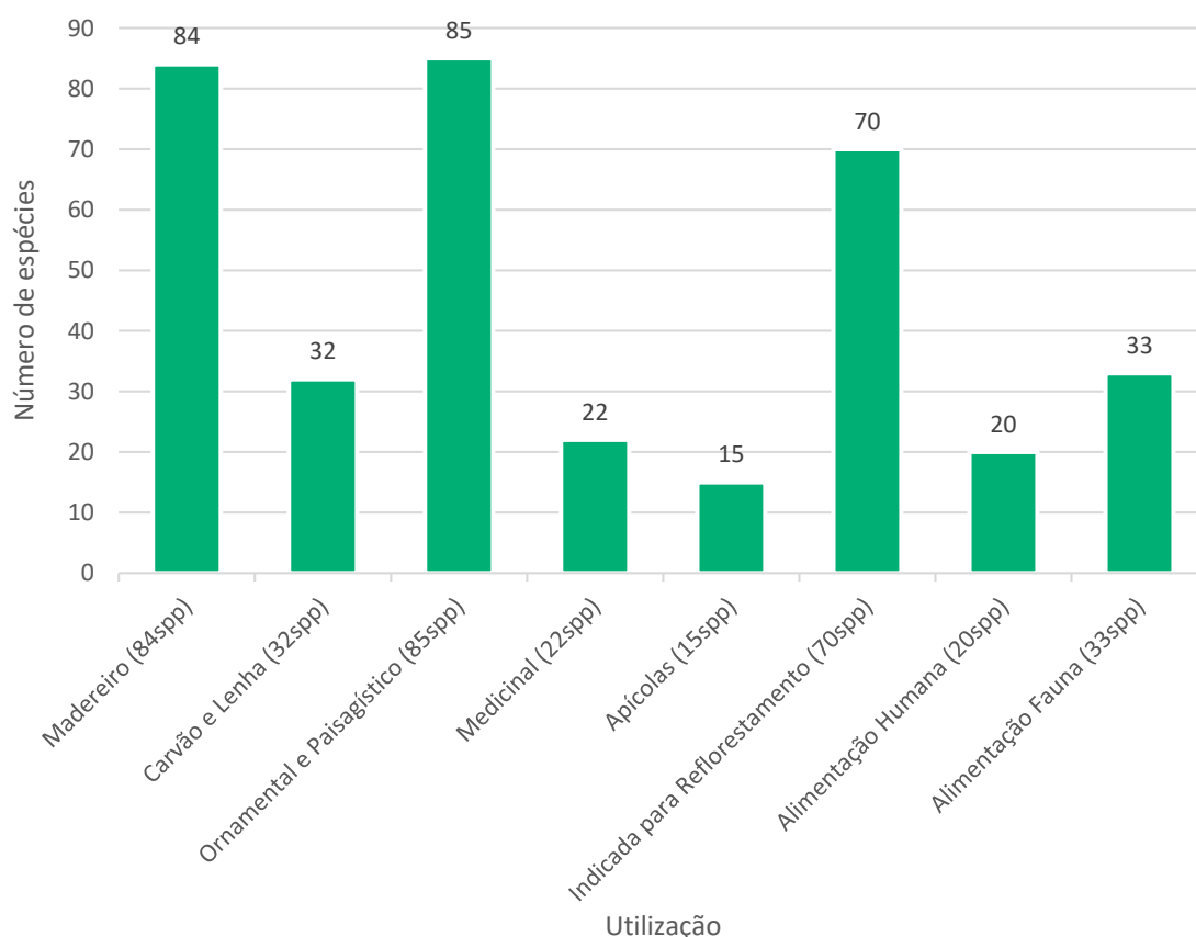
Gráfico 10.1-3: Número de espécies dentro de cada classe de uso.
