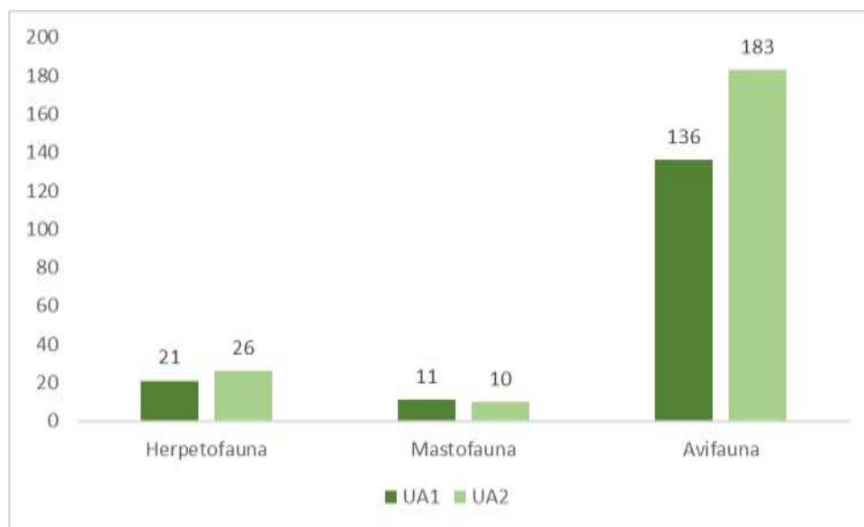
Gráfico 10.1-31: Riqueza da fauna por unidade amostral obtida a partir de coleta de dados primários (1ª e 2ª campanha).
