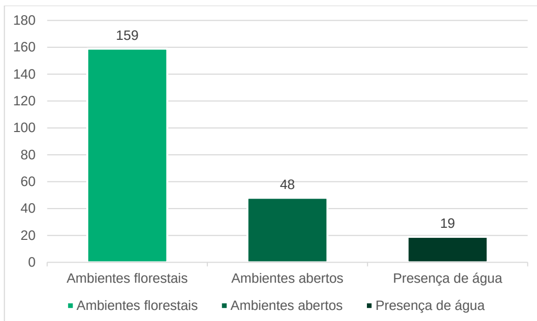
Gráfico 10.1-24: Gráfico representativo do número de espécies por ambiente preferencial para o grupo Avifauna.
