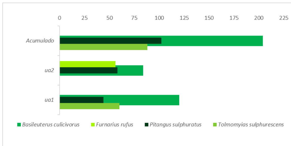
Gráfico 10.1-19: Espécies mais abundantes de aves por Unidade Amostral e acumulada obtida a partir do método de Censo Pontual de Abundância de Indivíduos e Espécie na área do empreendimento.
