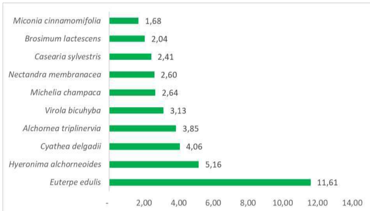
Gráfico 10.1-10: As dez espécies com maior Valor de Importância (VI%) no presente estudo.
