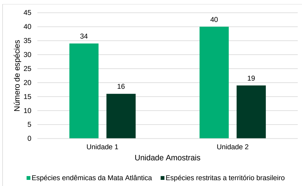
Gráfico 10.1-23: Gráfico comparativo das Unidades Amostrais quanto ao número de espécies de aves com algum tipo de distribuição restrita.
