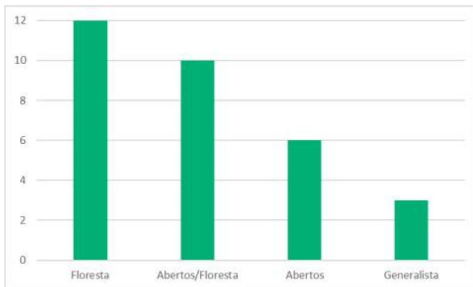
Gráfico 10.1-16: Habitat preferencial da herpetofauna registrada na área de influência do a LT 525/230 kV Rio do Sul – Indaial – Gaspar II.
