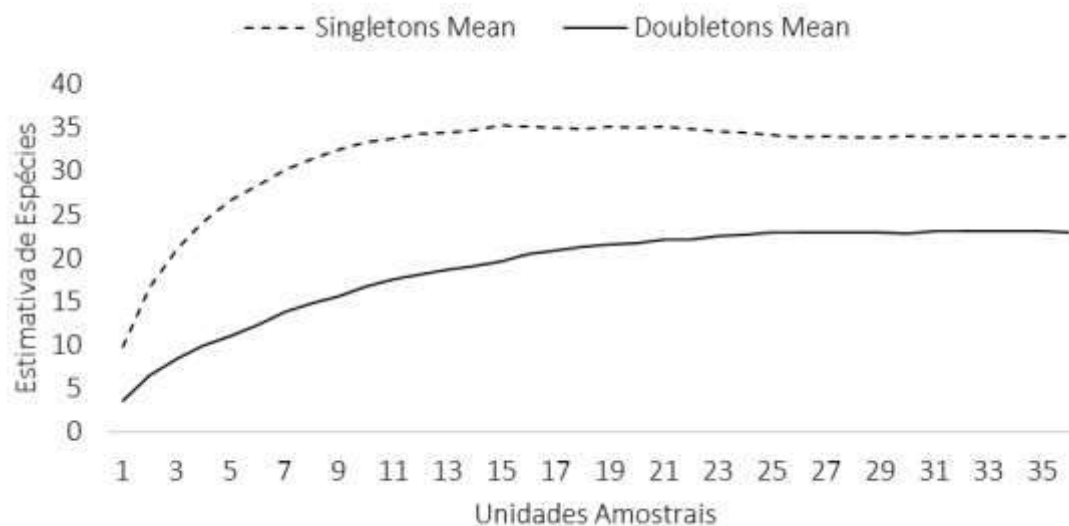
Gráfico 10.1-7: Gráfico com Singleton (um indivíduo nas amostras) e Doubleton (número de espécies com apenas dois indivíduos nas amostras).
