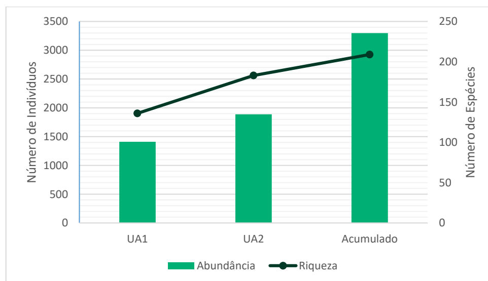
Gráfico 10.1-18: Riqueza e abundância do grupo Avifauna por Unidade Amostral e acumulada obtida a partir do método de Censo Pontual de Abundância de Indivíduos e Espécie na área do empreendimento.
