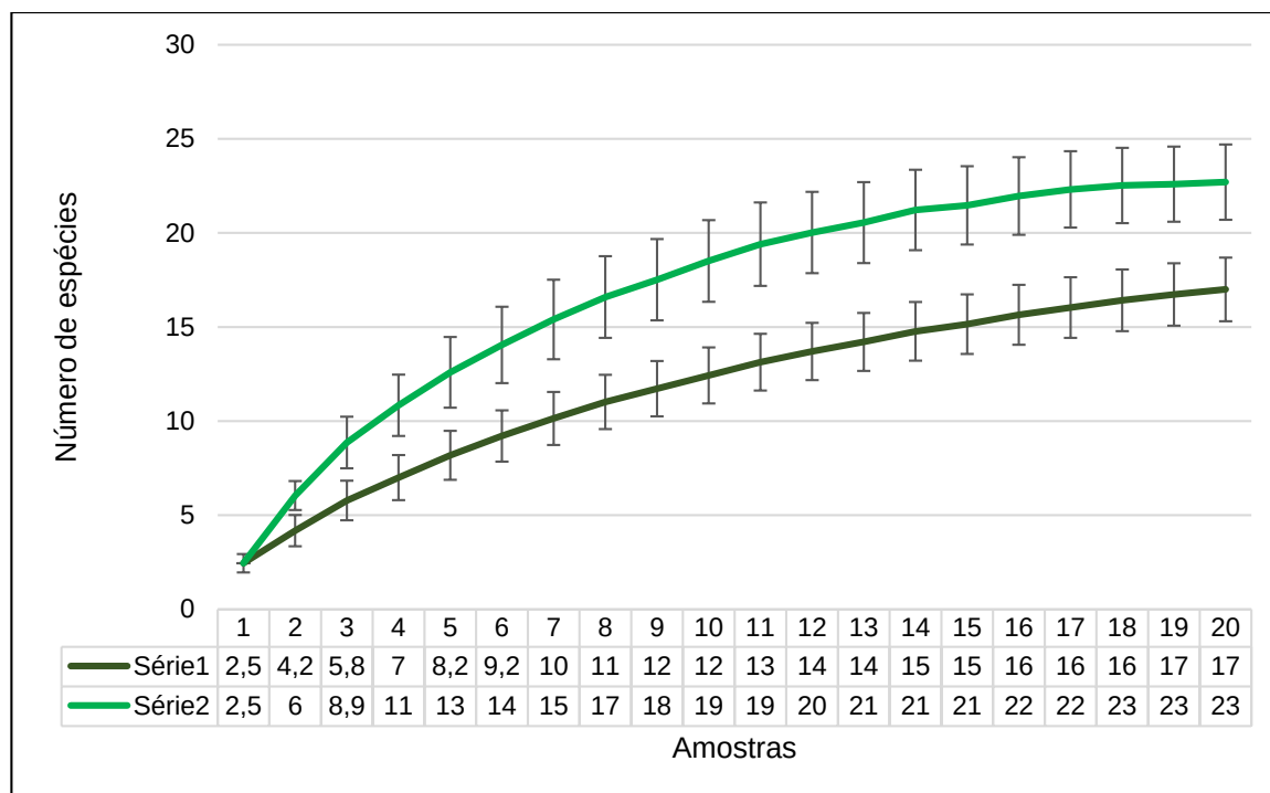
Gráfico 10.1-29: Curva do Coletor/ Rarefação da mastofauna na área de influência do empreendimento (campanha de verão e outono de 2019).
