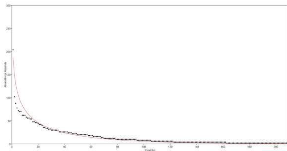
Gráfico 10.1-20: Curva da componente dominância para o grupo Avifauna.
