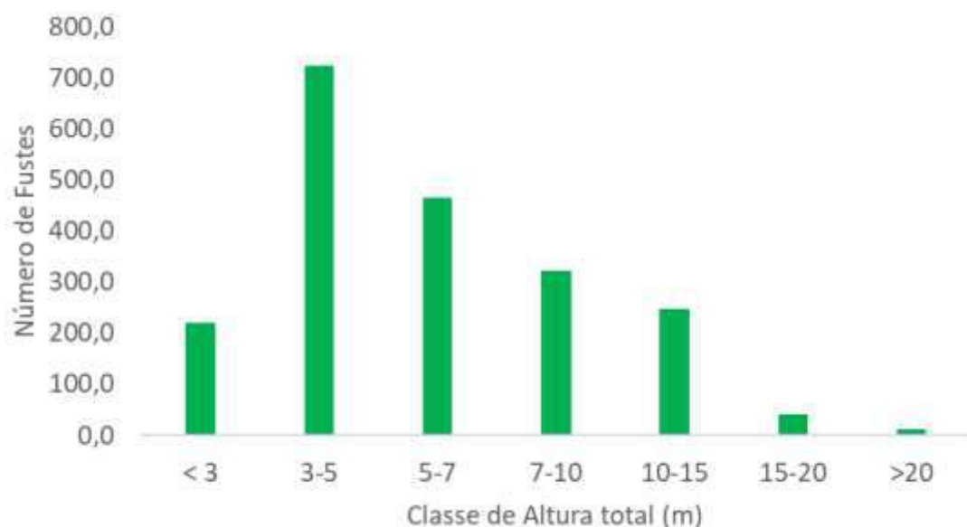
Gráfico 10.1-9: Distribuição por classe de altura total.
