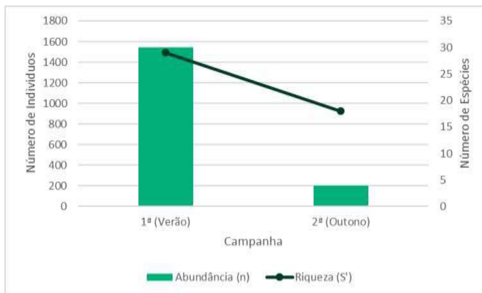
Gráfico 10.1-17: Abundância e Riqueza obtidas a partir do levantamento de campo de anfíbios e répteis do empreendimento.
