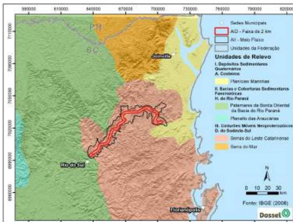
Figura10.1-11: Detalhe do Mapa "Unidade de Relevo do Brasil" com a localização da área de estudo. Fonte: (IBGE (2006).
