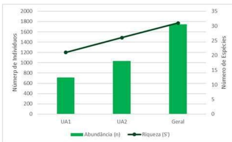
Gráfico 10.1-30: Abundância e Riqueza obtidas a partir do levantamento de campo de mamíferos.
