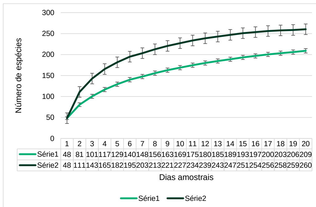
Gráfico 10.1-22: Curva do Coletor Rarefação da avifauna na área de influência da LT 525/230 kV Rio do Sul – Indaial – Gaspar II, Subestações e seccionamentos associados (campanha de verão e outono de 2019).
