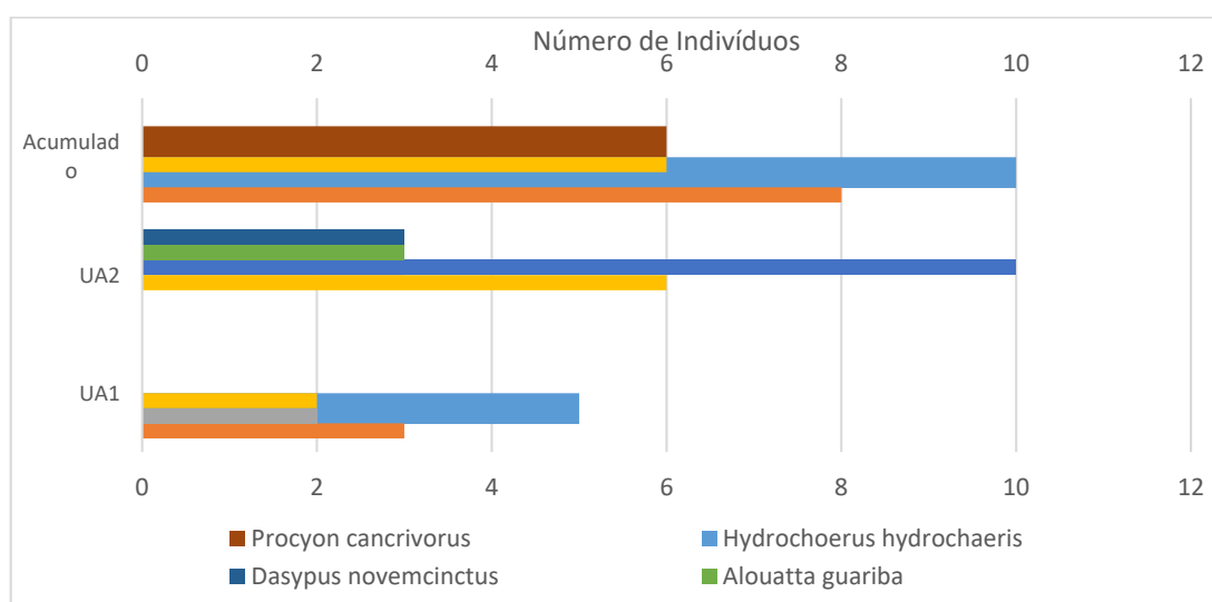
Gráfico 10.1-27: Espécies mais abundantes de mamíferos por Unidade Amostral e acumulada na área do empreendimento.
