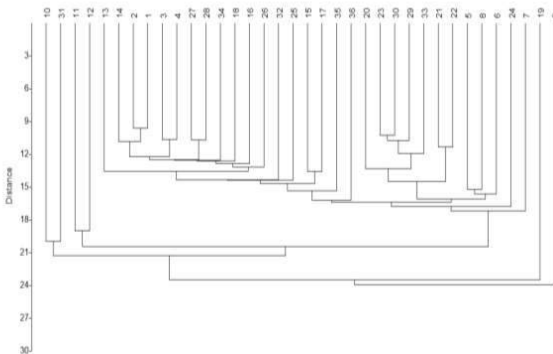
Gráfico 10.1-4: Gráfico de Distância Euclidiana atribuído as parcelas.
