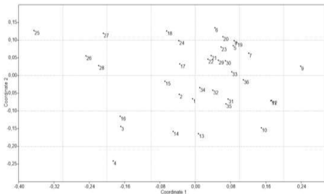
Gráfico 10.1-5: MDS obtido pela similaridade de Bray-Courts.
