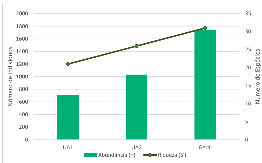
Gráfico 10.1-11: Riqueza e Abundância por Unidade Amostral e Acumulado da herpetofauna considerando as duas campanhas sazonais (verão e outono).
