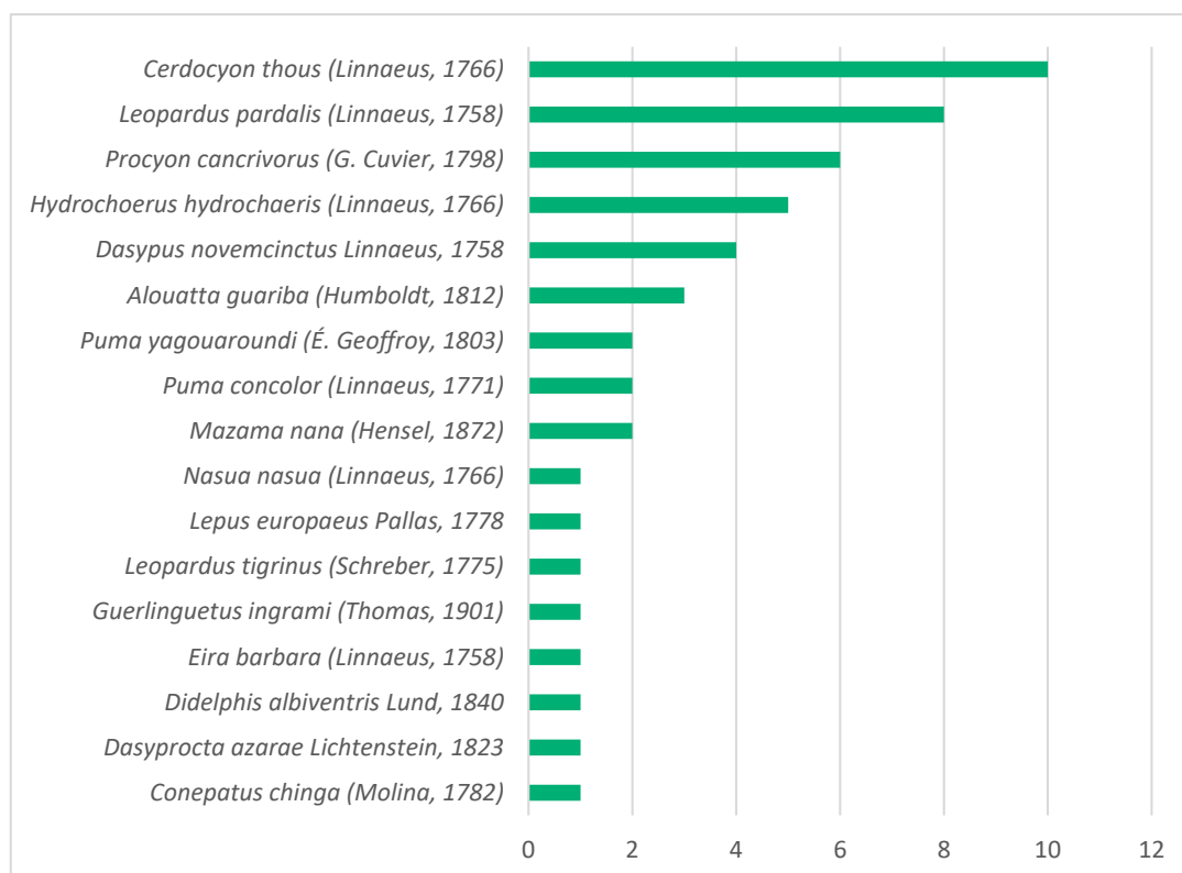
Gráfico 10.1-26: Abundância das espécies da mastofauna registradas na 1ª e 2ª campanha (verão e outono).
