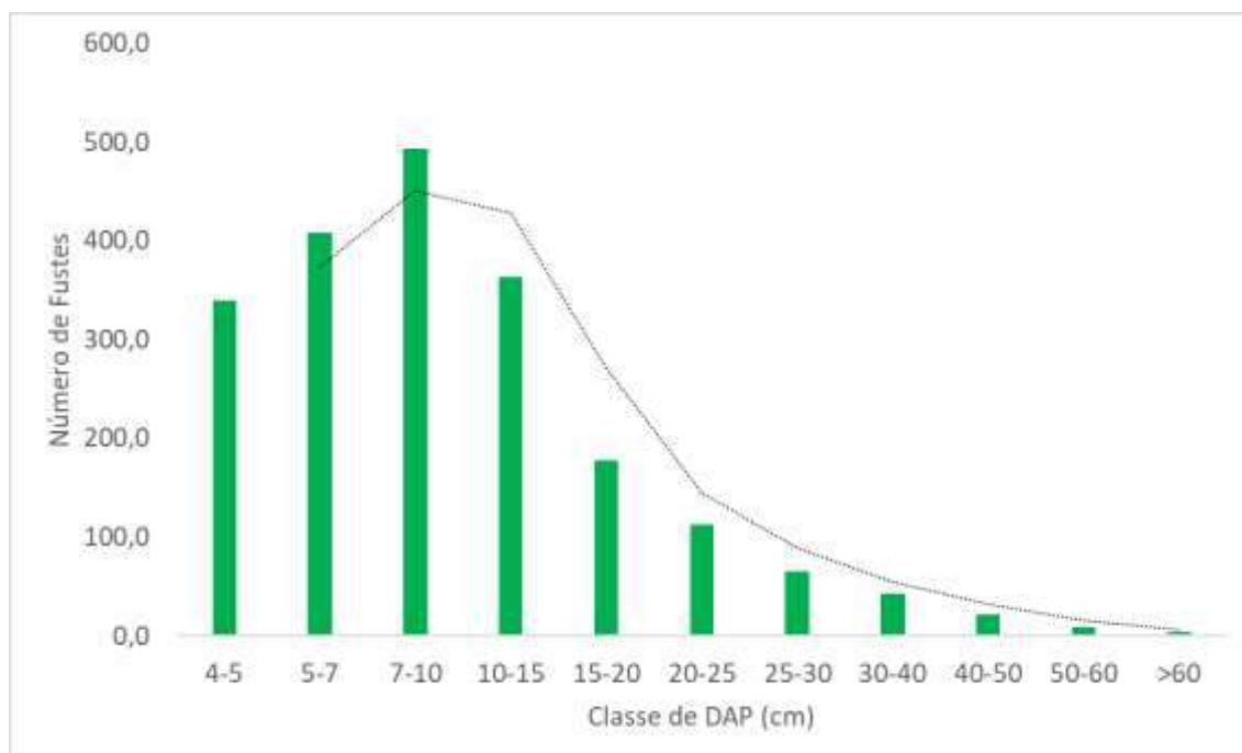
Gráfico 10.1-8: Distribuição por classe de DAP (Diâmetro a Altura do Peito).
