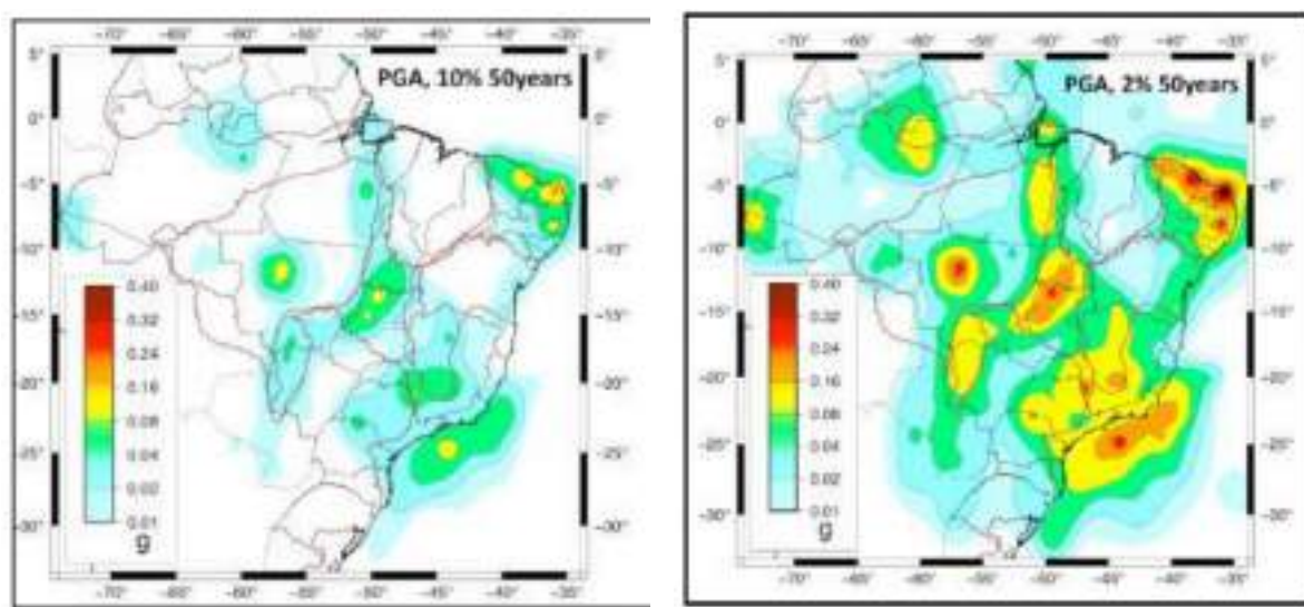
Figura 10.1-24: Mapas de Ameaça Sísmica (“Seismic Hazard Maps”) para aceleração de pico (PGA) em rocha, para probabilidades de 10% (a) e 2% (b) de excedência em 50 anos, correspondendo a períodos de retorno de 475 e 1.475 anos, respectivamente. As cores são PGA em frações de g. Áreas verdes correspondem a PGA entre 4% e 8% g (equivalente a intensidades ~VI na escala Mercalli Modificada, podendo causar trincas em paredes), áreas amarelas entre 8% e 16% g (intensidades ~VII MM podendo causar rachaduras em paredes e desabamento de casas fracas). ” Fonte: ASSUMPÇÃO (2016).
