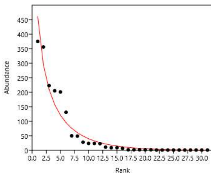
Gráfico 10.1-13: Curva de dominância do grupo Herpetofauna.
