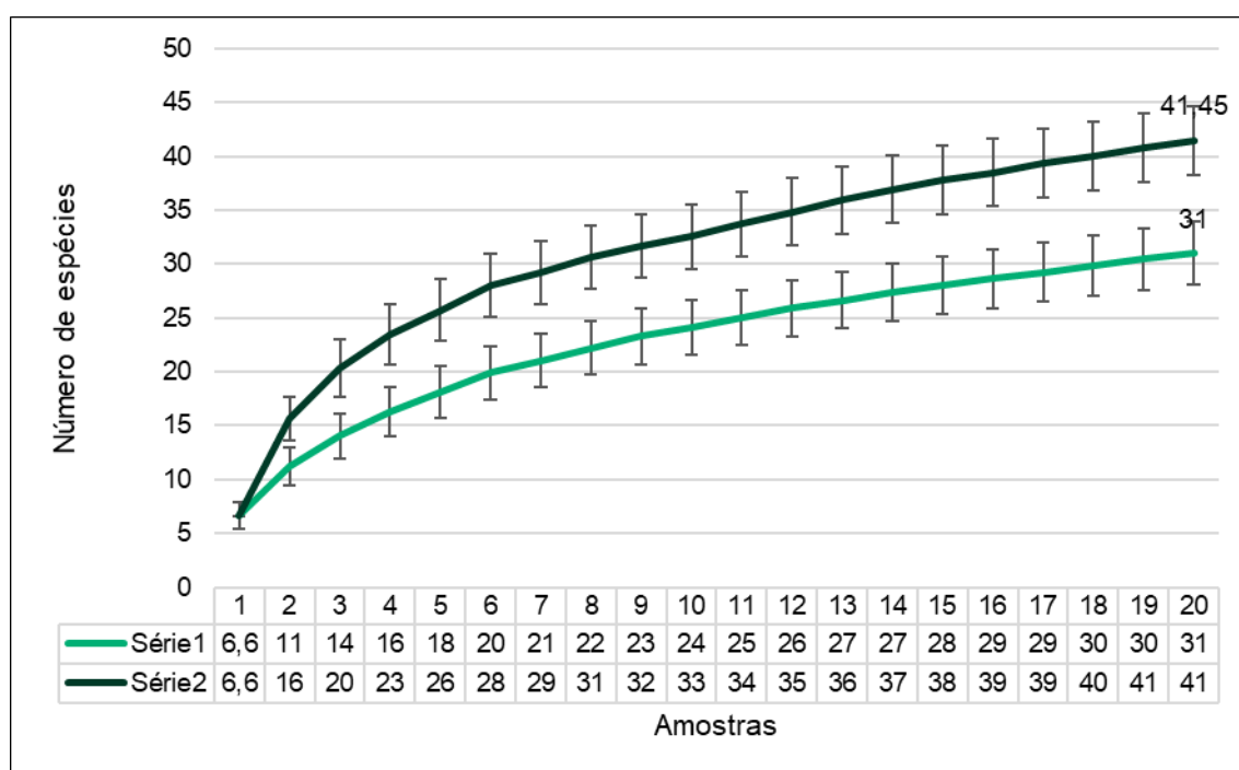
Gráfico 10.1-15: Curva do Coletor/ Rarefação dos anfíbios e répteis na área de influência (campanhas de verão e outono de 2019).
