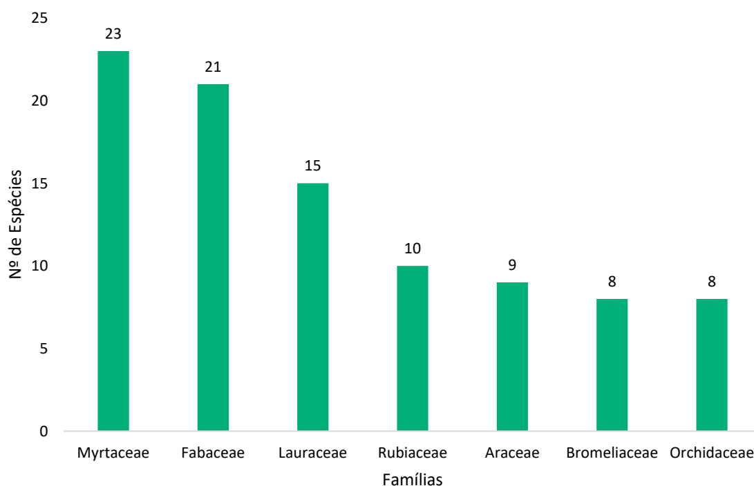
Gráfico 10.1-1: Riqueza de espécies das Famílias Botânicas mais representativas da área de estudo.
