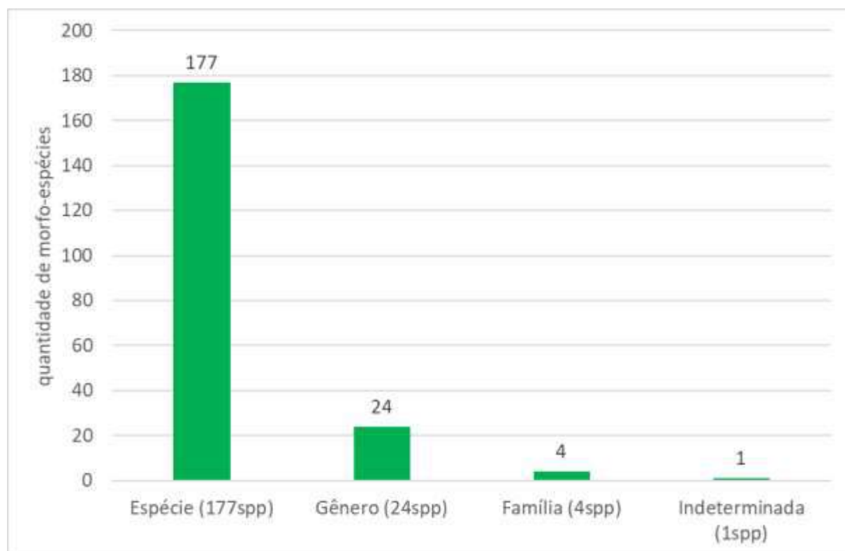
Gráfico 10.1-2: Eficácia de identificação no presente estudo.
