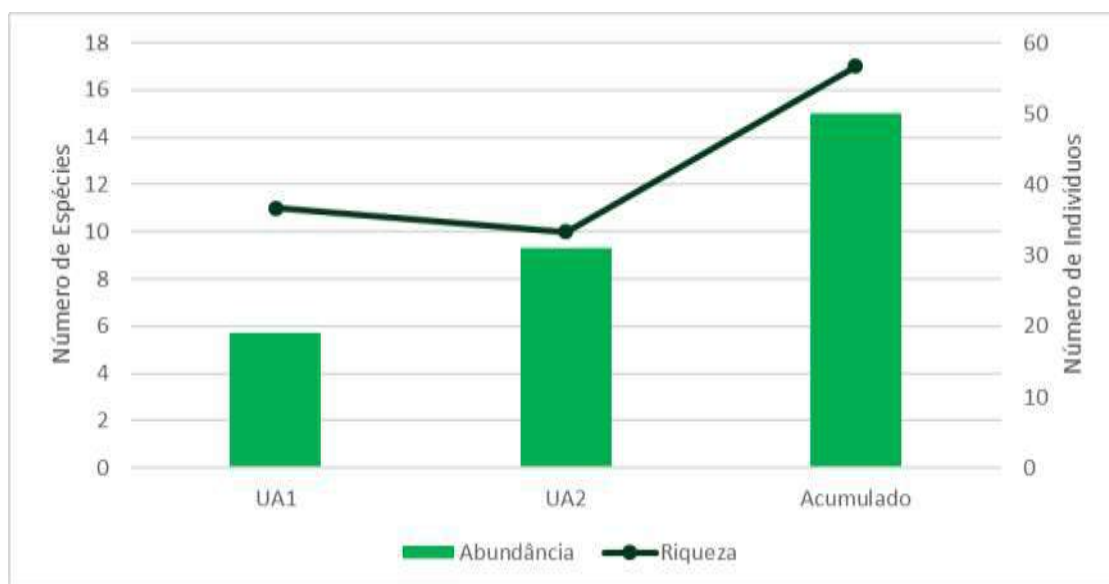
Gráfico 10.1-25: Riqueza e abundância do grupo mastofauna por Unidade Amostral e acumulada na área do empreendimento.
