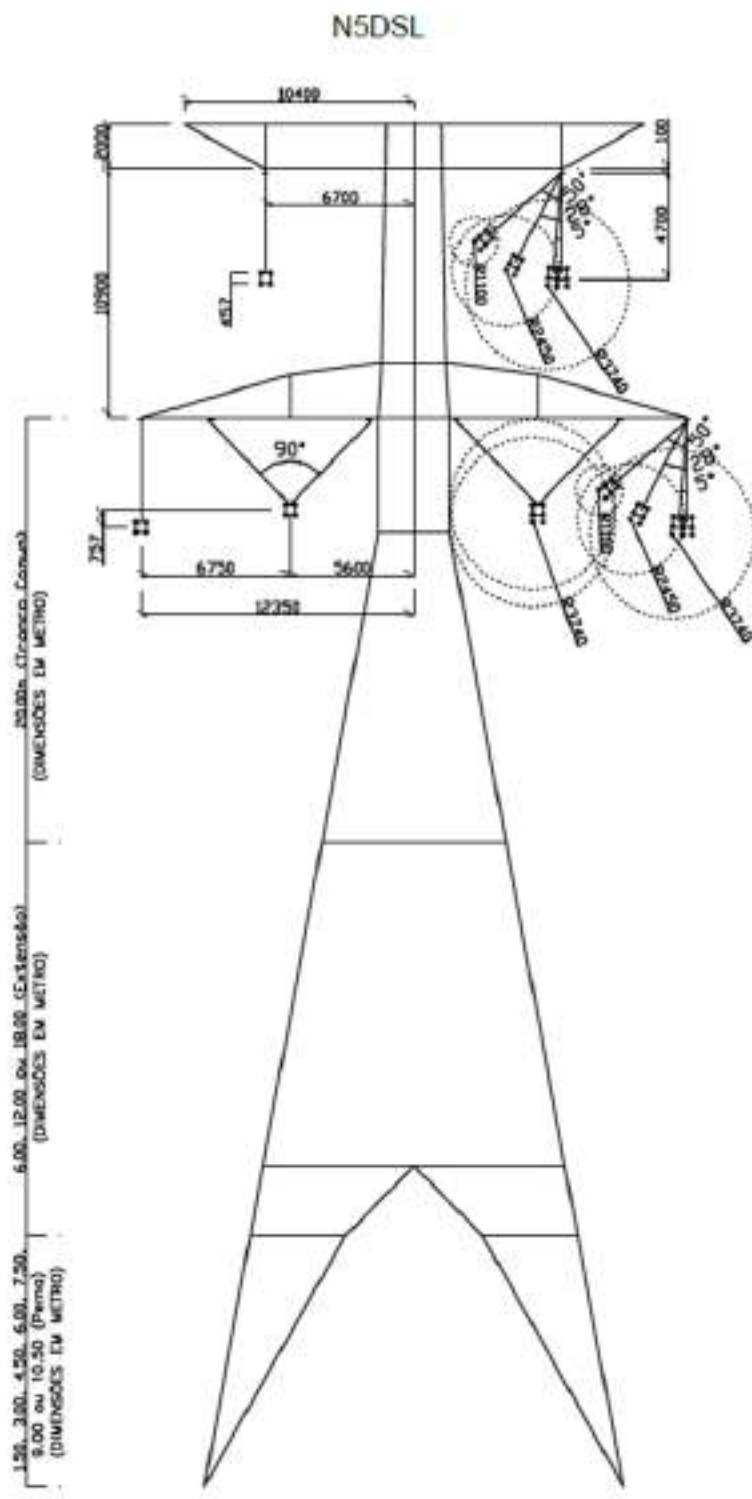
Figura 6.3-4: Silhueta da estrutura N5DSL (Torre Autoporte de Suspensão Leve) LT de 525 kV.
