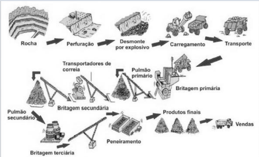
Fluxograma do processo produtivo relacionado as atividades minerárias no local.
